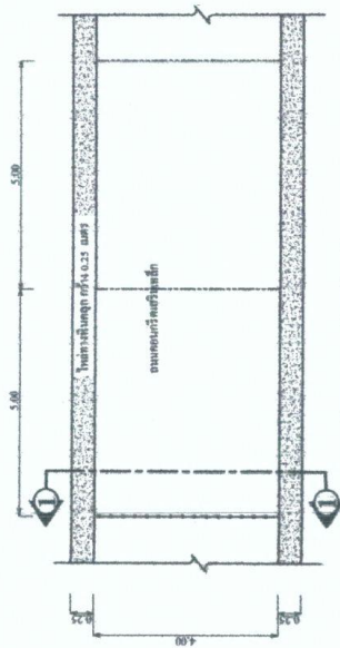
แผ่นคอนกรีตเสริมเหล็ก ขนาด 5.00 ม. x 0.25 ม. อัตราส่วน 1 : 100
